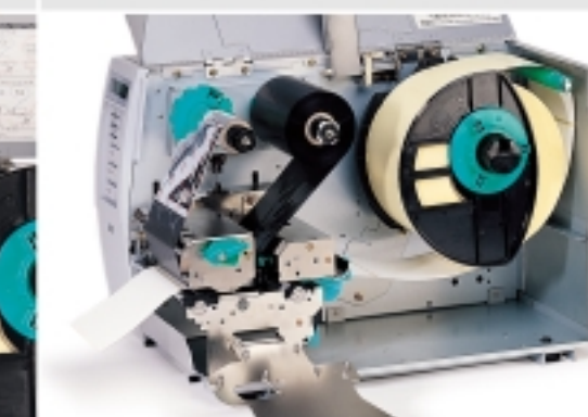
▲ Un mécanisme qui s'ouvre largement.
