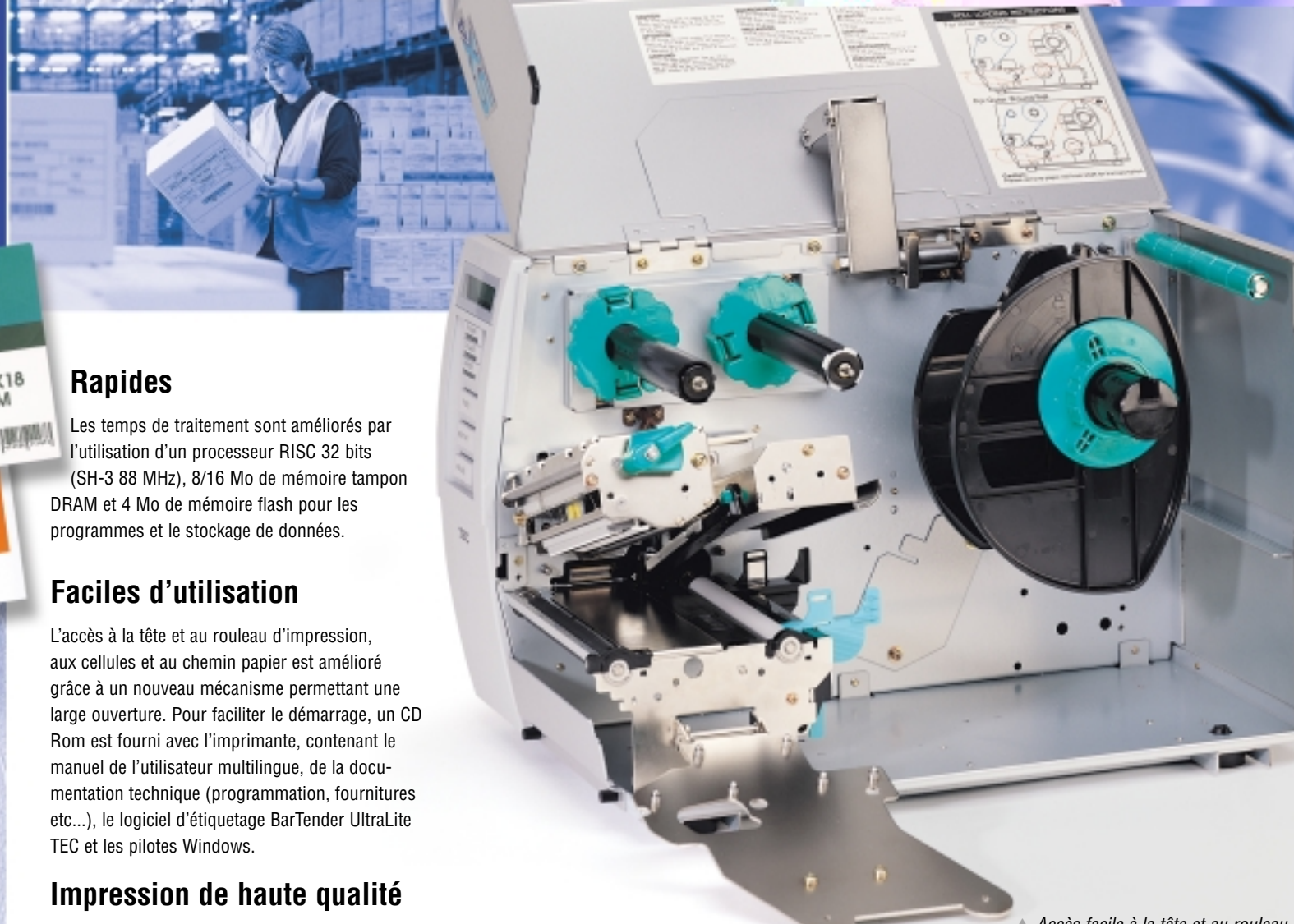
▲ Accès facile à la tête et au rouleau d'impression, aux cellules et au chemin papier.
